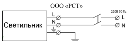
Рис. 1 Схема подключения светильника
